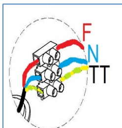
Figura 3 (Conexión eléctrico)
